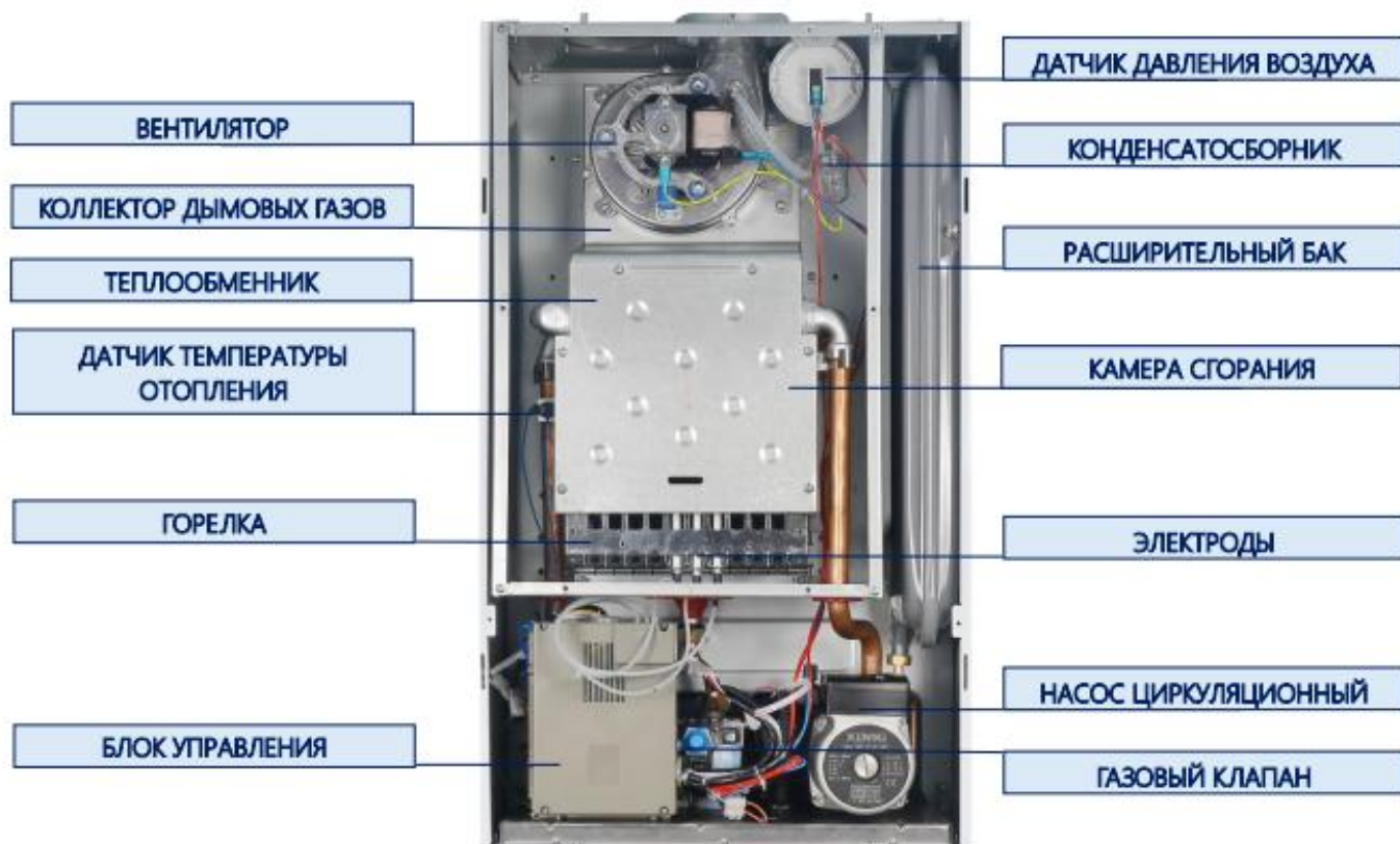
Рисунок 2. Строение котла.
