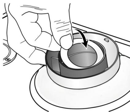
Рисунок 5. Диафрагма дымохода
