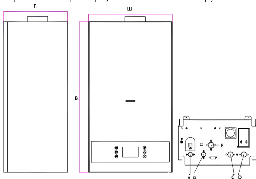
Рисунок 1. Размеры корпуса и обозначение патрубков котлов
