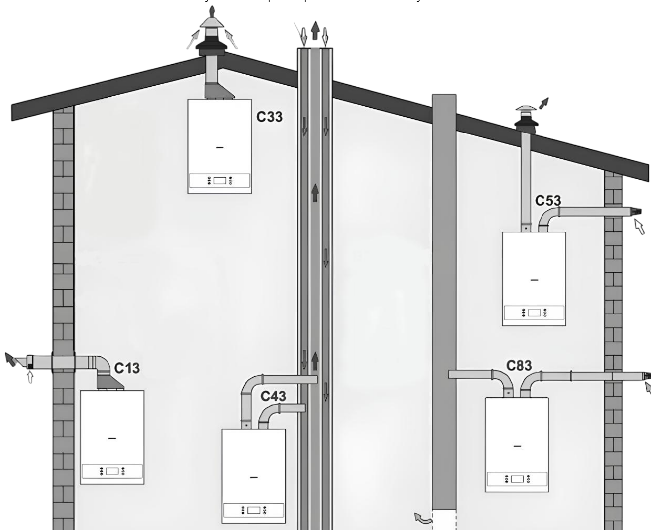
Рисунок 7. Примеры систем дымоудаления
