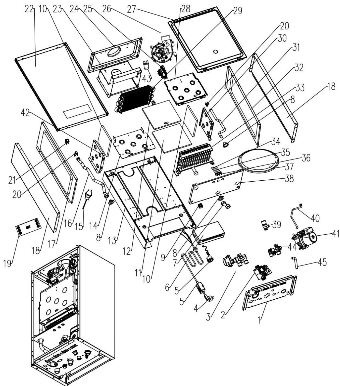
Рисунок 3. Взрывная схема котлов
