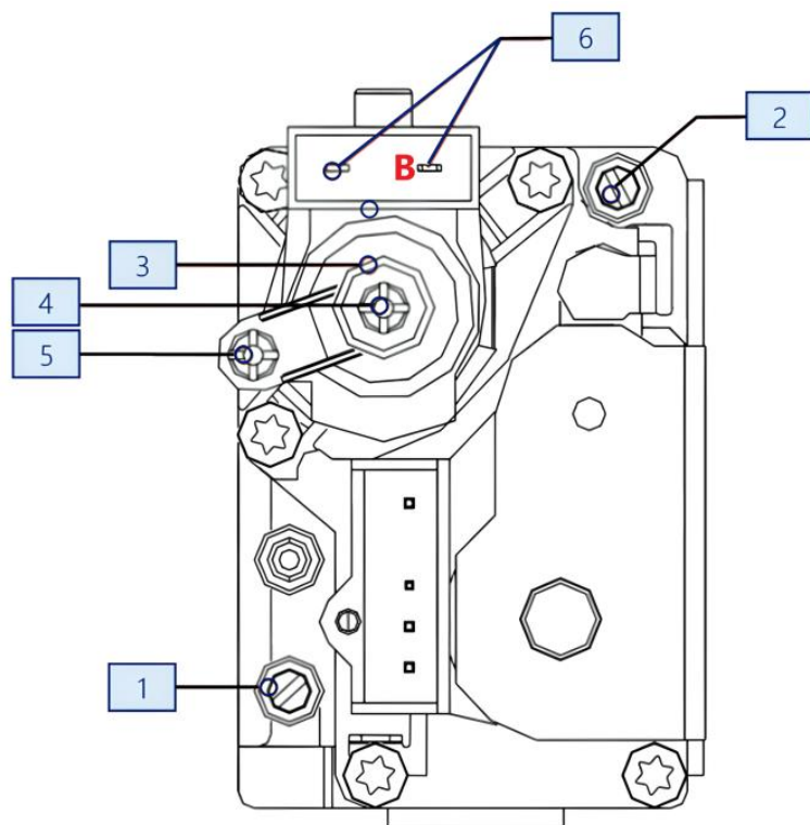
Рисунок 8. Газовый клапан
