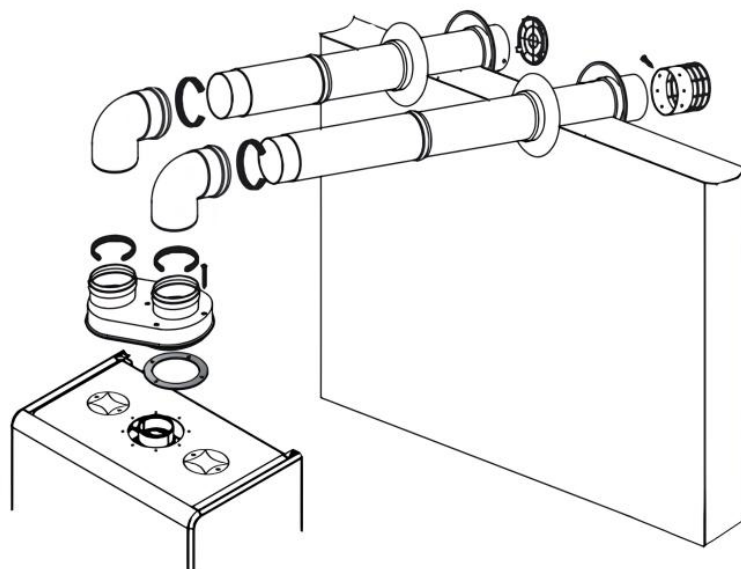
Рисунок 6. Подключение адаптера раздельного дымохода
