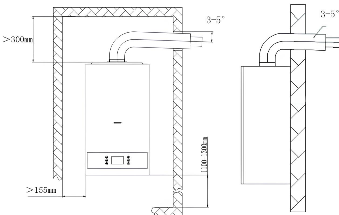
Рисунок 4. Установка котла
